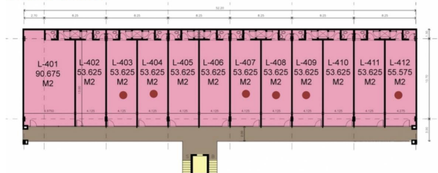
PLANTA 4to. NIVEL
